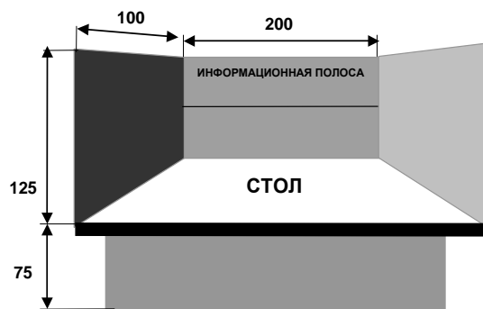
СХЕМА ВЫСТАВОЧНОГО СТЕНДА (размеры указаны в см)
